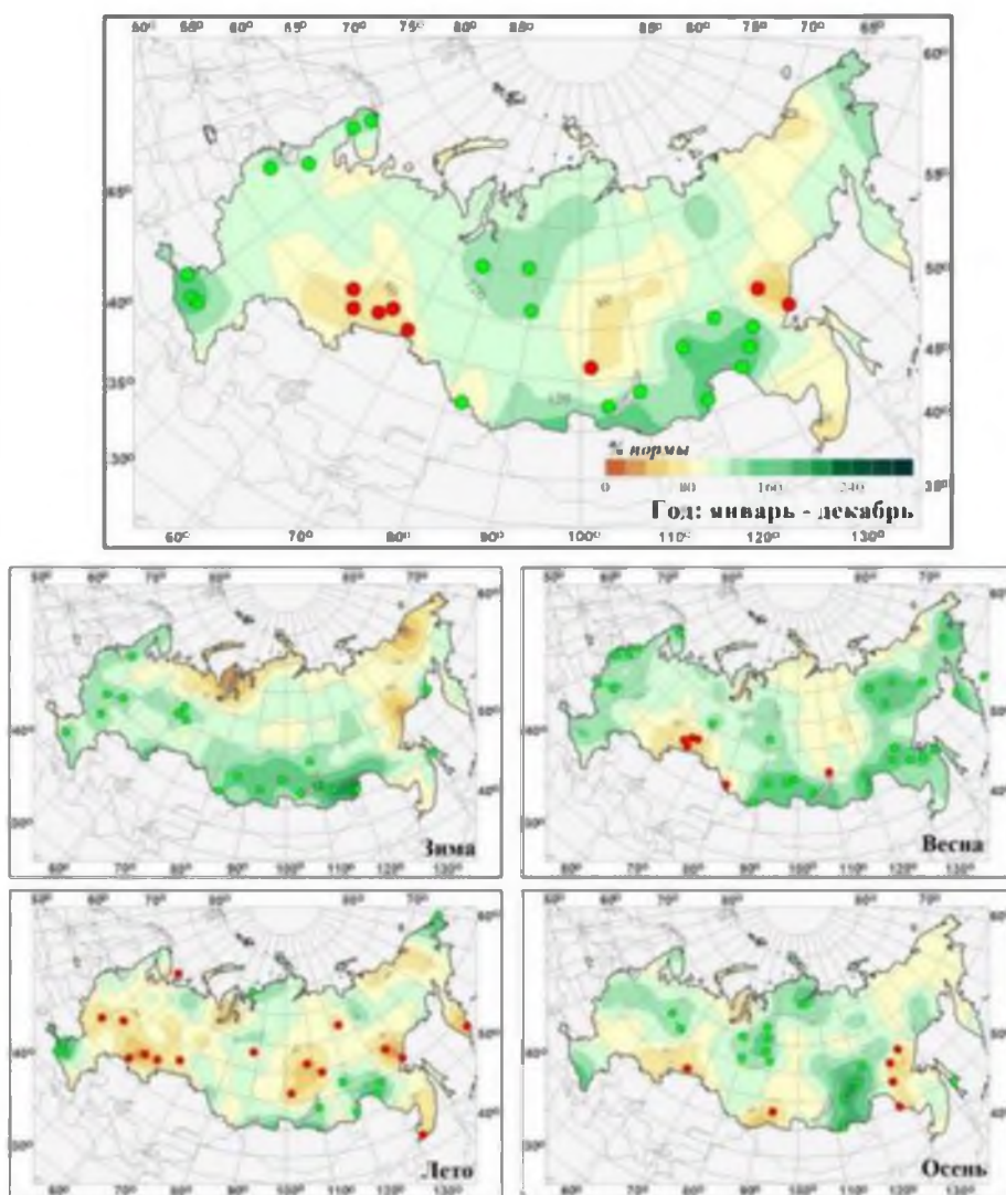
Рисунок 6.1.2 – Аномалии осадков на территории России в 2021 г., с указанием локализации 5%-х экстремумов (красные кружки) и 95%-х (зеленые кружки)
