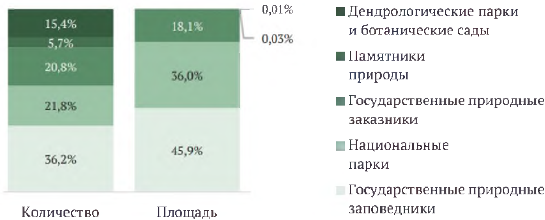
Рисунок 6.7.2 – Соотношение количества и площади ООПТ федерального значения в 2021 г.
